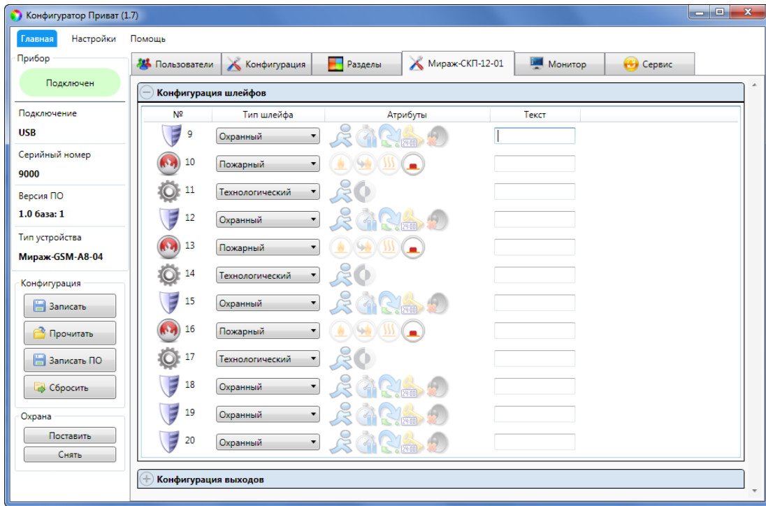
Рисунок 7.49 – Блок Конфигурация шлейфов СКП
