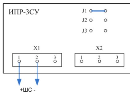
Рисунок 6.6 — Подключение извещателя ИПП-ЗСУ с имитацией дымового извещателя
